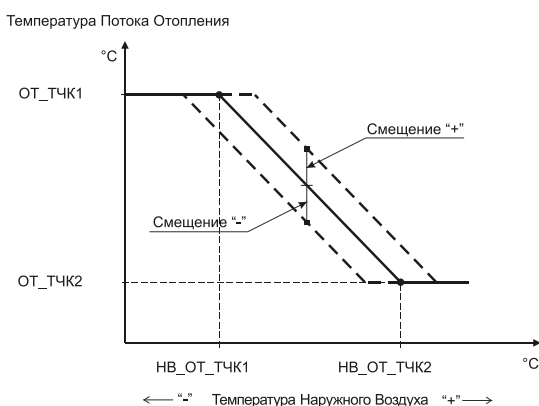
График Расчетной Уставки Темп. Поточка Отопления со Смещением
