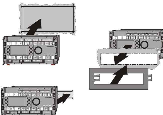
Рис. 2. Варианты монтажа
