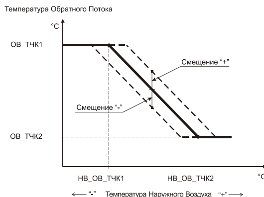
График Расчетной Уставки Темп. Обратного Потoka со Смещением
